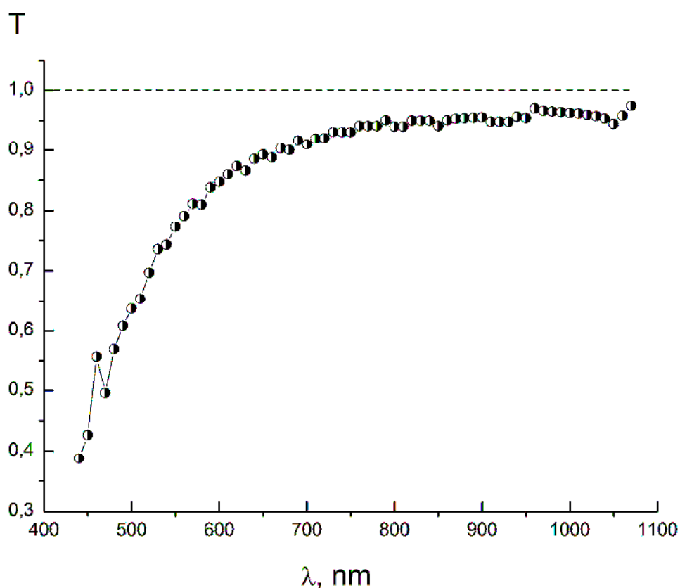
Рис. 3. Спектральная зависимость коэффициента пропускания, определяющаяся как отношение величины оптического сигнала прошедшего через исследуемый экстракт и растворитель. Спектр получен при температуре 293 К
