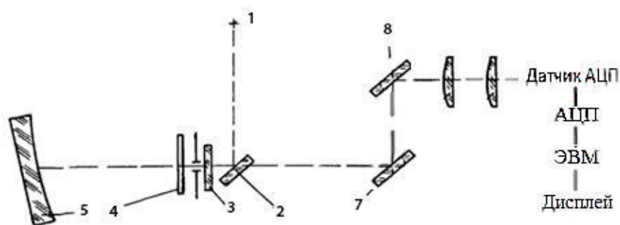
Рис. 1. Оптическая и электронно-информационная схема спектрофотометра СФ-46. Основные элементы: 1 – источник света, 2 – поворотное зеркало, 3 – щель, 4 – светофильтр, 5 – дифракционная решетка, 7 – образец, 8 – зеркало
