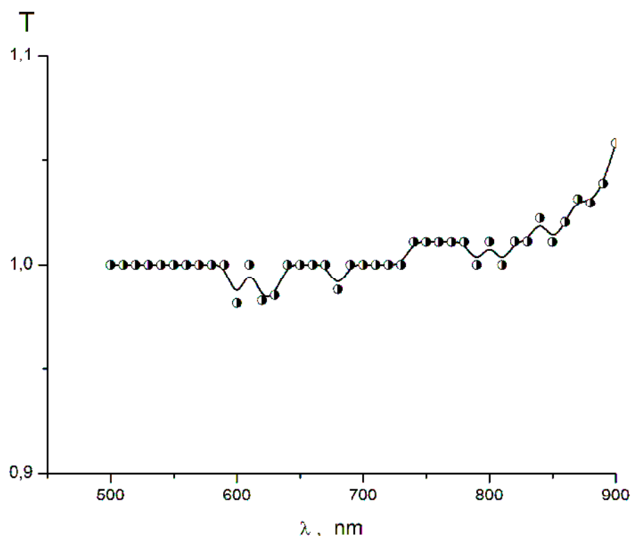
Рис. 2. Спектр пропускания растворителя на основе водного раствора этилового спирта с толщиной слоя 10 мм при температуре 293 К
